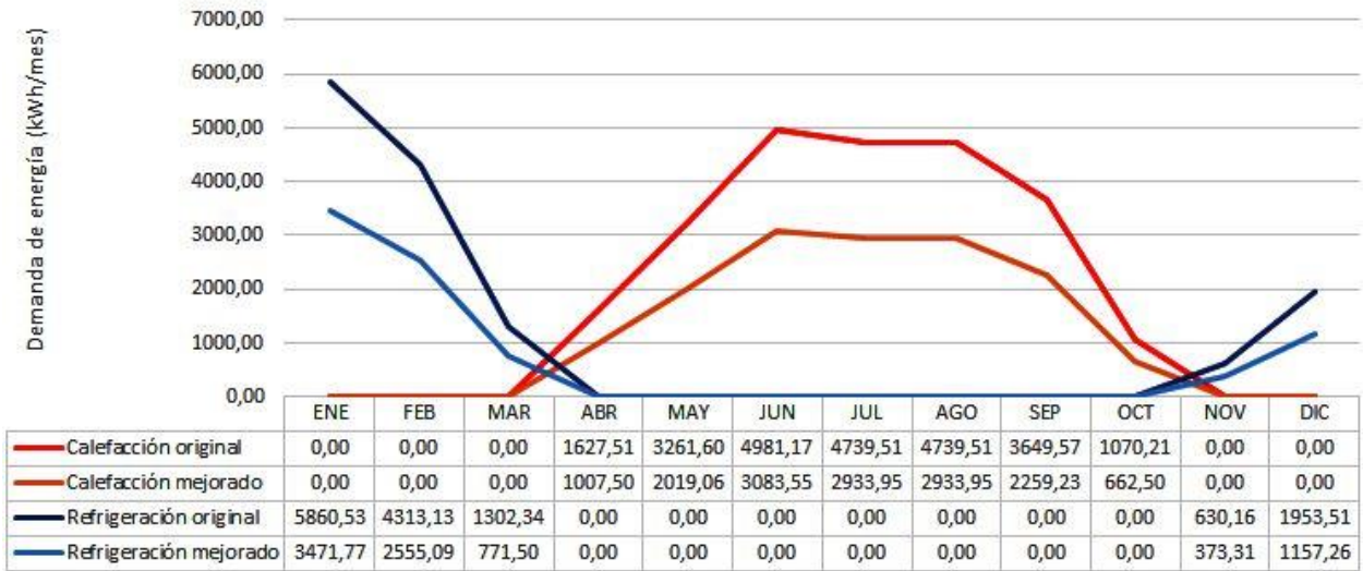
Figura 11: Comparación anual. caso: Biblioteca Municipal de Tapalqué. Prov. De Buenos Aires.
