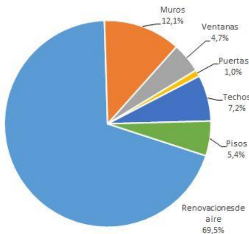
Figura 3: Pérdidas térmicas discriminadas situación mejorada
