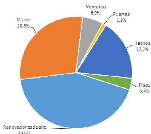
Figura 1: Pérdidas térmicas discriminadas situación original
