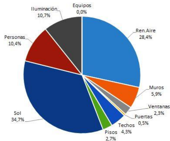
Figura 8: Aportes térmicos discriminados. Situación mejorada verano.
