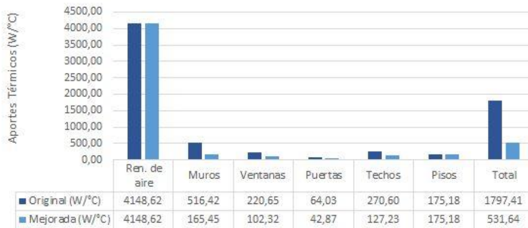
Figura 9: Comparación de edificio original y mejorado. Situación verano.
