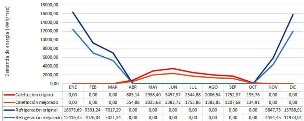
Figura 11: Comparación anual caso: Jardín de Infantes, Soldini, Santa Fe.
