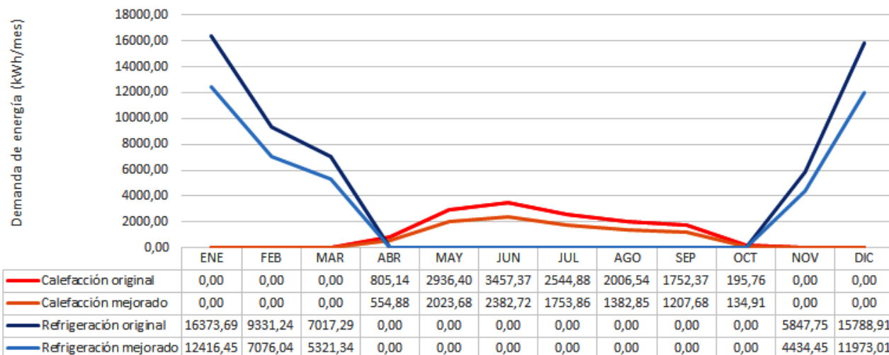
Figura 1: Comparación de demandas de energía en climatización mensual original y con mejoras.
