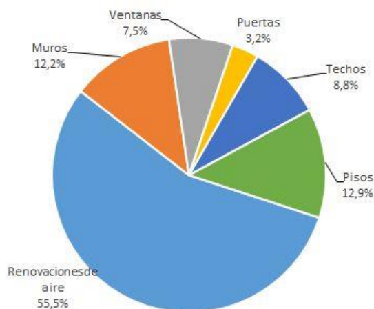
Figura 3: Pérdidas térmicas discriminadas situación mejorada
