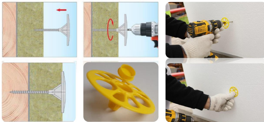
Fijación prevista para edificios con H < 10 m 6 fijaciones/m 2 en el centro 6 fijaciones/m 2 en las esquinas
