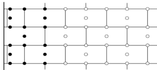
Fijación prevista para edificios con H < 10 m 6 fijaciones/m 2 en el centro 6 fijaciones/m 2 en las esquinas
