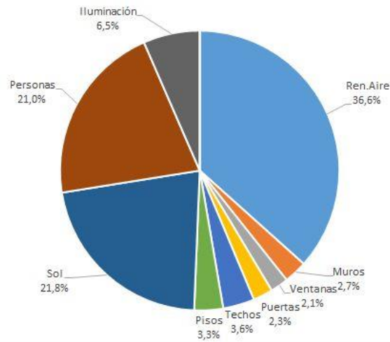
Figura 8: Aportes térmicos discriminados. Situación mejorada verano.
