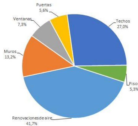
Figura 1: Pérdidas térmicas discriminadas situación original
