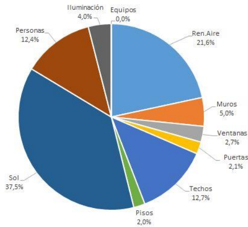
Figura 6: Aportes térmicos discriminados. Situación original verano.
