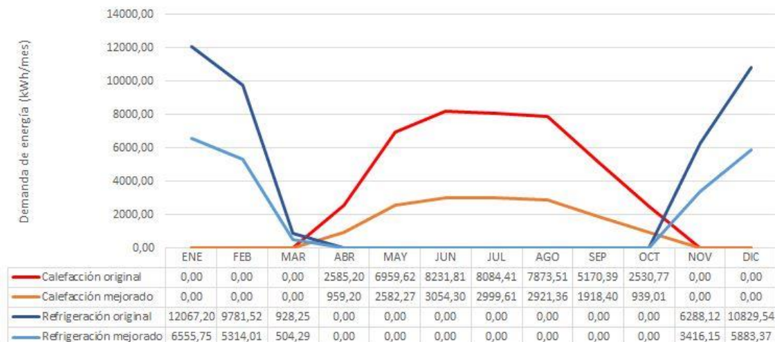
Figura 11: Comparación anual caso: Jardín maternal "Mariano Moreno", Neuquén. Neuquén.
