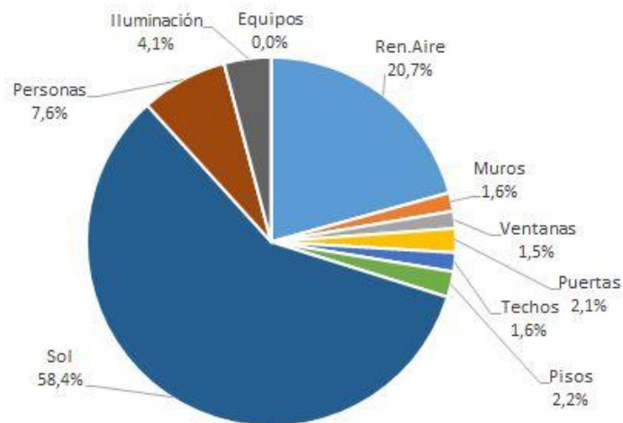
Figura 8: Aportes térmicos discriminados. Situación mejorada verano.
