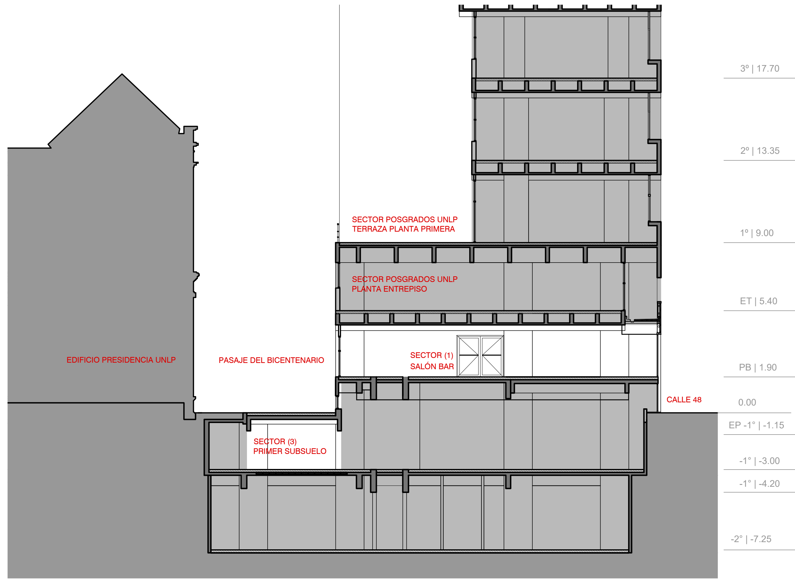
CORTE B-B
