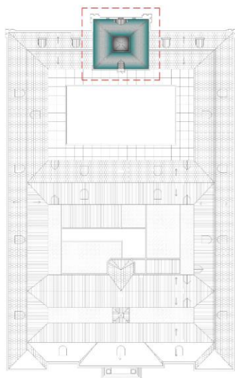
PLANTA Y CORTE EDIFICIO PRESIDENCIA – SECTOR CÚPULA
