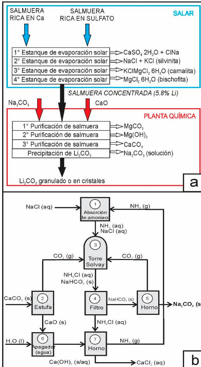
Figura 2. a. Obtencción de \text{Li}_2\text{CO}_3 a partir de salmuera en Salar de Atacama (Chile). Modificado de [5]. b. Proceso SOLVAY.
